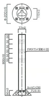
PF-N800-24 高さ 800mm ダイヤモンドグレート反射シート3枚 スタンダードタイプ 接着剤目安: 300g (排水性舗装: 360g)
